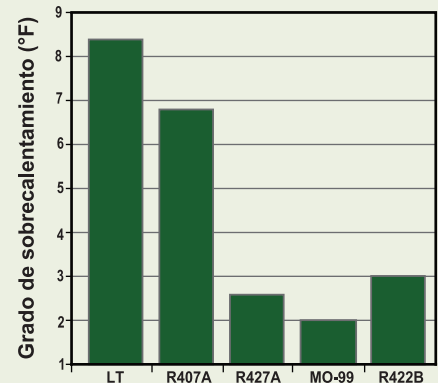
Figura 2. En un análisis de reemplazo directo, Genetron Performax LT preserva el sobrecalentamiento, protegiendo los compresores y asegurando el uso eficiente de la capacidad del refrigerante.
