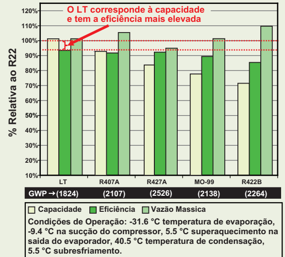
Figura 1. O Genetron Performax LT supera as alternativas disponíveis para novas instalações em supermercados e suas modernizações
