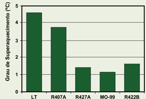
Figura 2. O Genetron Performax LT preserva o grau de superaquecimento, protegendo os compressores e garantindo o uso total da capacidade de refrigeração.
